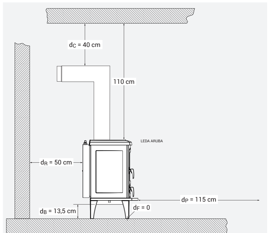
ARUBA: Mindestabstände zu brennbaren Materialien – schematische Darstellung mit oberem Anschluss, Seitenansicht
