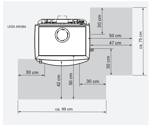
ARUBA: Nicht brennbarer Belag vor den Feuerraumöffnungen – schematische Darstellung
