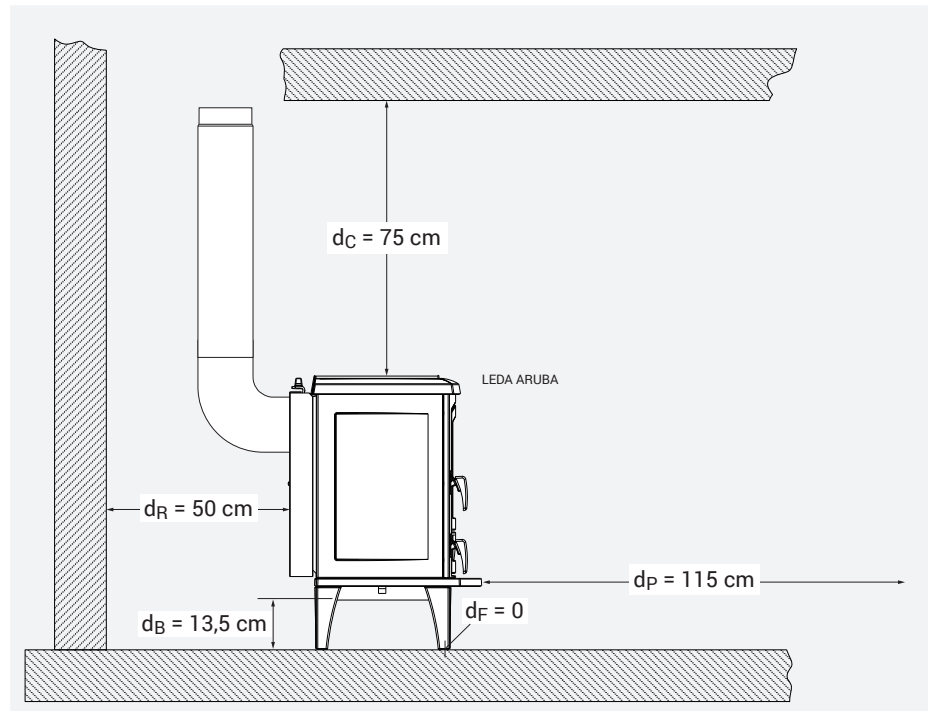
ARUBA: Mindestabstände zu brennbaren Materialien – schematische Darstellung mit hinterem Anschluss, Seitenansicht
