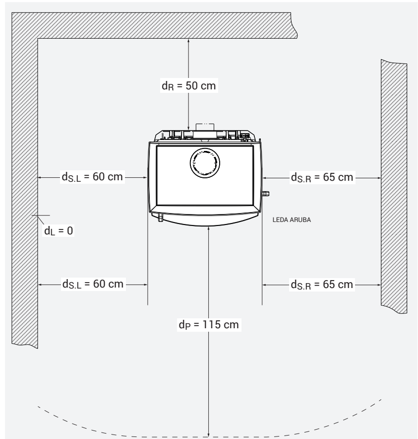
ARUBA: Mindestabstände zu brennbaren Materialien
