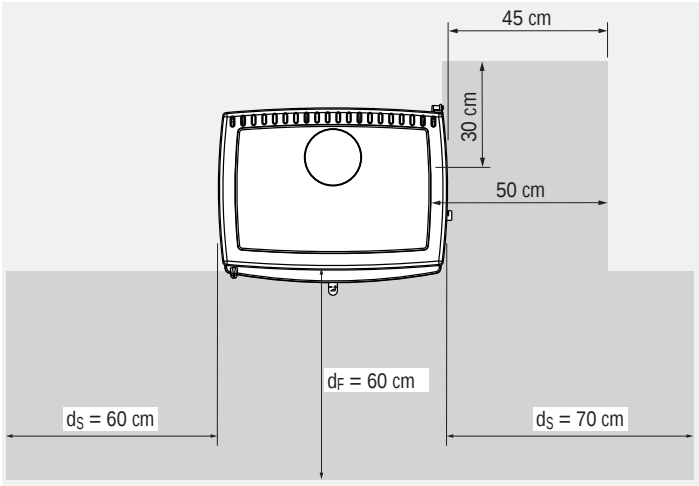
Abb. 2.6 ALLEGRA: Nicht brennbarer Belag vor den Feuerraumöffnungen – schematische Darstellung
