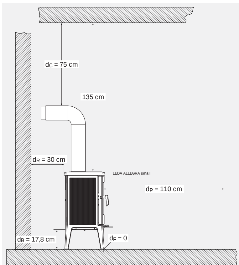
Abb. 2.4 ALLEGRA small: Mindestabstände zu brennbaren Materialien – schematische Darstellung, Seitenansicht
