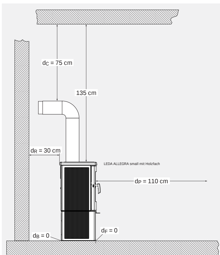
Abb. 2.5 ALLEGRA small mit Holzfach: Mindestabstände zu brennbaren Materialien – schematische Darstellung, Seitenansicht
