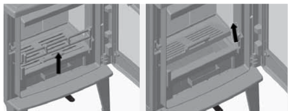
Abb. 4.20 Entnehmen des Stehrosts und Bodenrosts
