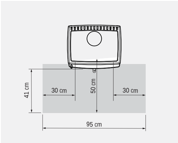
Abb. 2.8 ALLEGRA small oder ALLEGRA small mit Holzfach: Nicht brennbarer Belag vor der Feuerraumöffnung – schematische Darstellung
