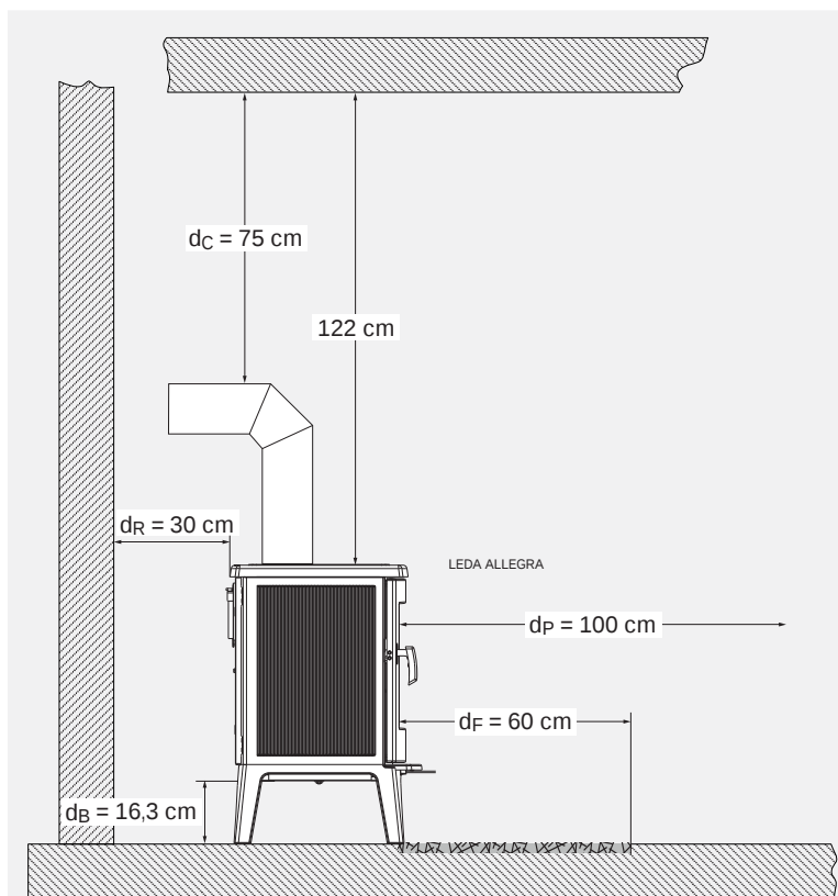
Abb. 2.3 ALLEGRA: Mindestabstände zu brennbaren Materialien – schematische Darstellung, Seitenansicht
