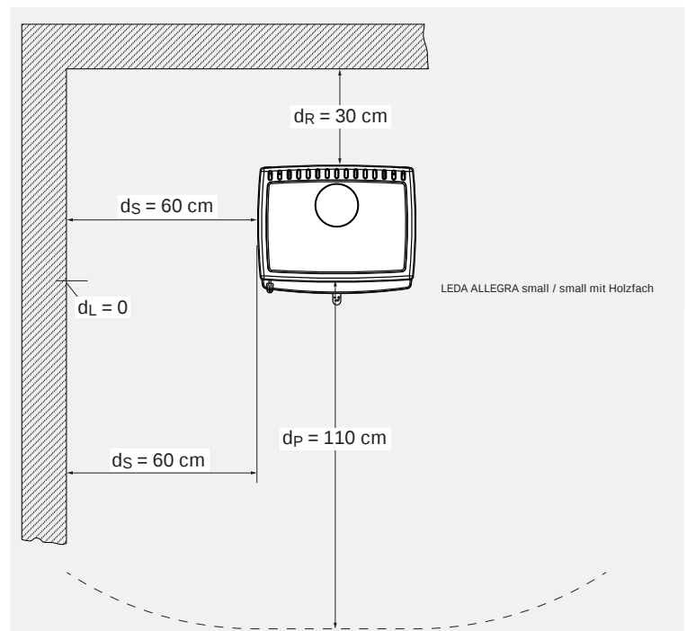
Abb. 2.2 ALLEGRA small oder ALLEGRA small mit Holzfach: Mindestabstände zu brennbaren Materialien
