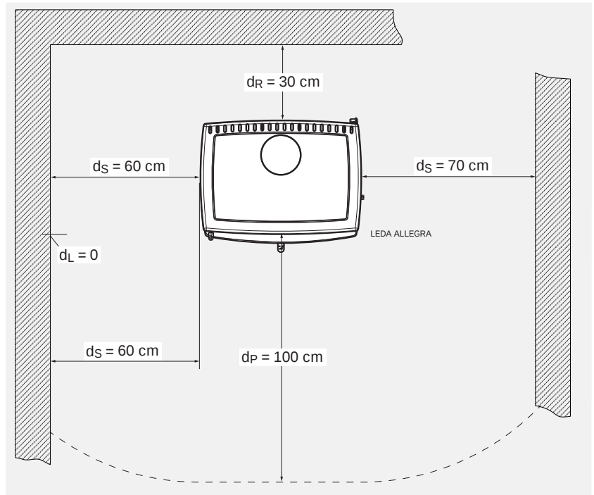
Abb. 2.1 ALLEGRA: Mindestabstände zu brennbaren Materialien
