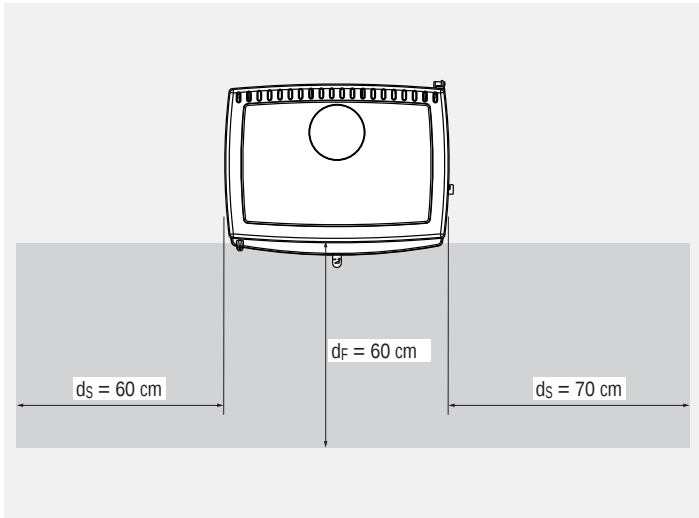
Abb. 2.7 ALLEGRA: Nicht brennbarer Belag vor der Feuerraumöffnung bei eingesetzter Türsicherung in der seitlichen Befülltür – schematische Darstellung
