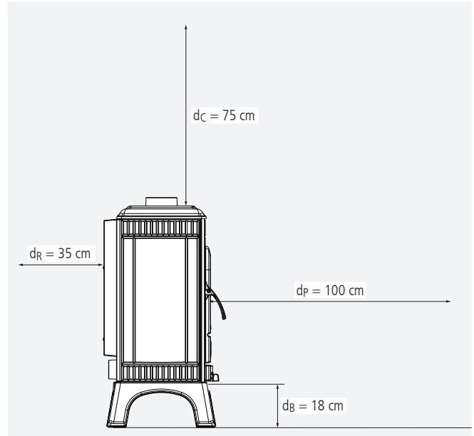
EDDA small: Mindestabstände zu brennbaren Materialien – schematische Darstellung, Seitenansicht
