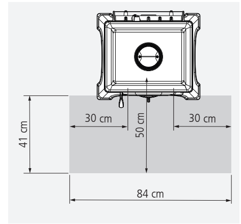
EDDA: Nicht brennbarer Belag vor der Feuerraumöffnung – schematische Darstellung
