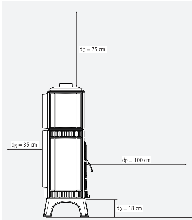
EDDA plus oder EDDA tea: Mindestabstände zu brennbaren Materialien – schematische Darstellung, Seitenansicht
