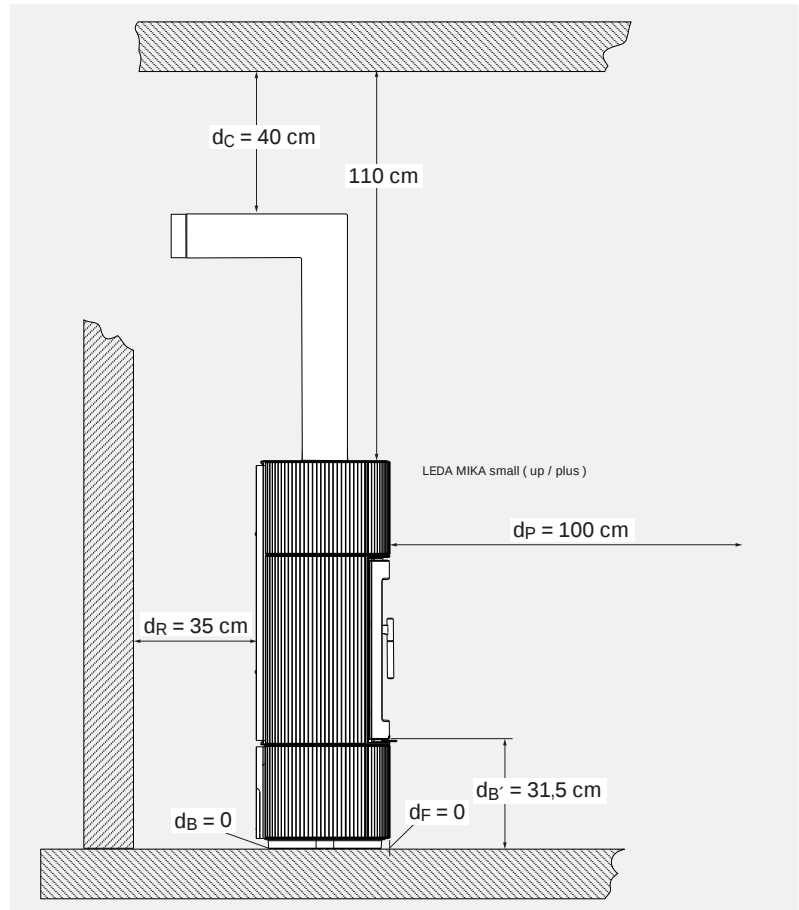
Abb. 2.3 MIKA: Strahlungsbereich der Sichtscheibe – schematische Darstellung, Seitenansicht
