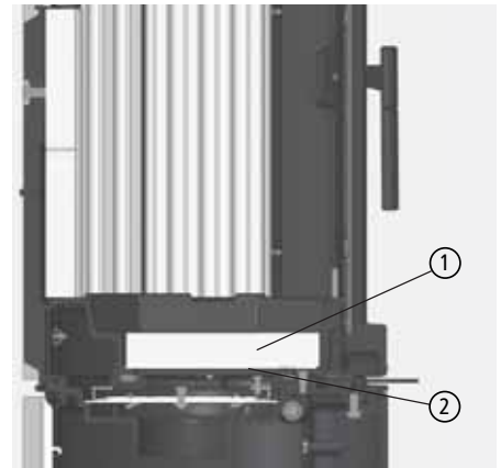
Abb. 4.35 Bodenstein, Bodenblech entnehmen
