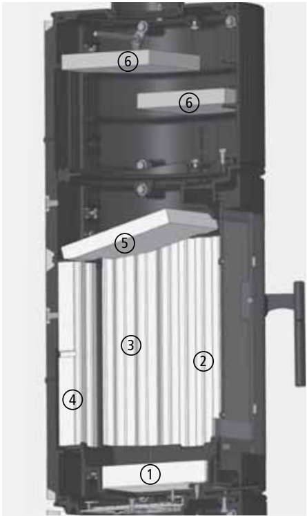
Abb. 5.1 Feuerraum-Auskleidung, Prallplatte, Umlenkungen
