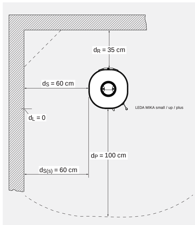
Abb. 2.1 MIKA: Mindestabstände zu brennbaren Materialien
