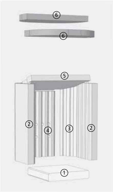
Abb. 5.2 Feuerraum-Auskleidung, Prallplatte und Umlenkung
