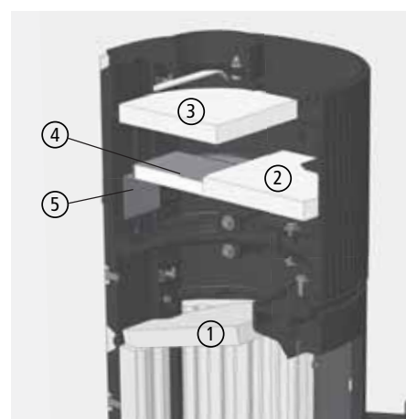
Abb. 4.39 Lage der Umlenkungen mit eingesetztem Katalysator
