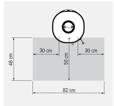
Abb. 2.4 MIKA: Nicht brennbarer Belag vor der Feuerraumöffnung – schematische Darstellung
