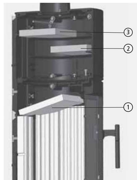
Abb. 4.38 Lage der Umlenkungen
