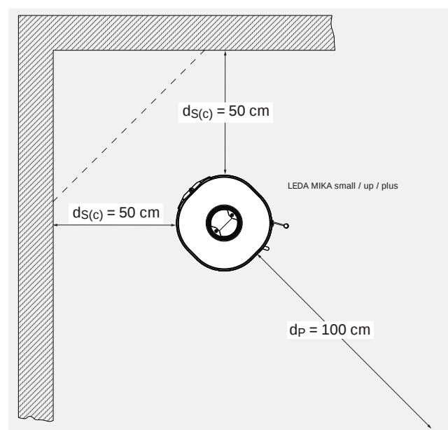
Abb. 2.2 MIKA: Mindestabstände zu brennbaren Materialien bei „Eckaufstellung“
