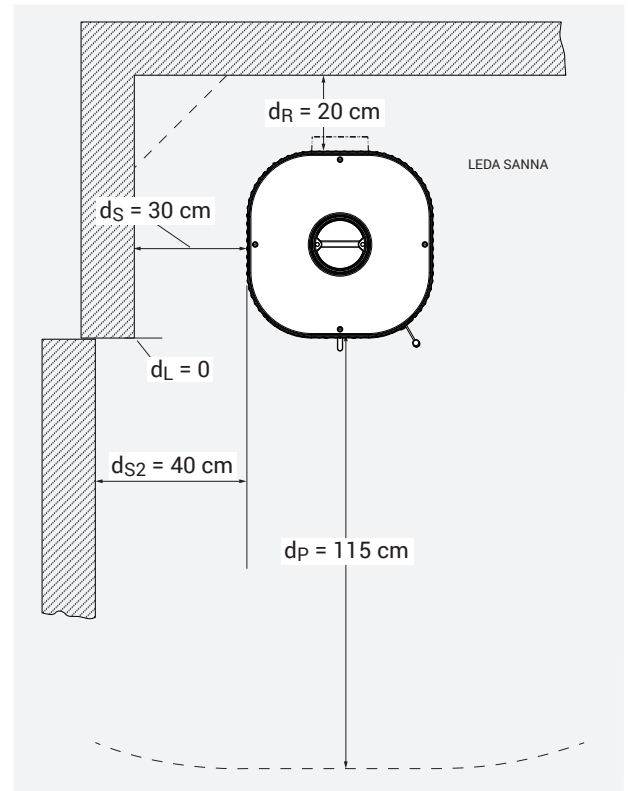
SANNA: Mindestabstände zu brennbaren Materialien
